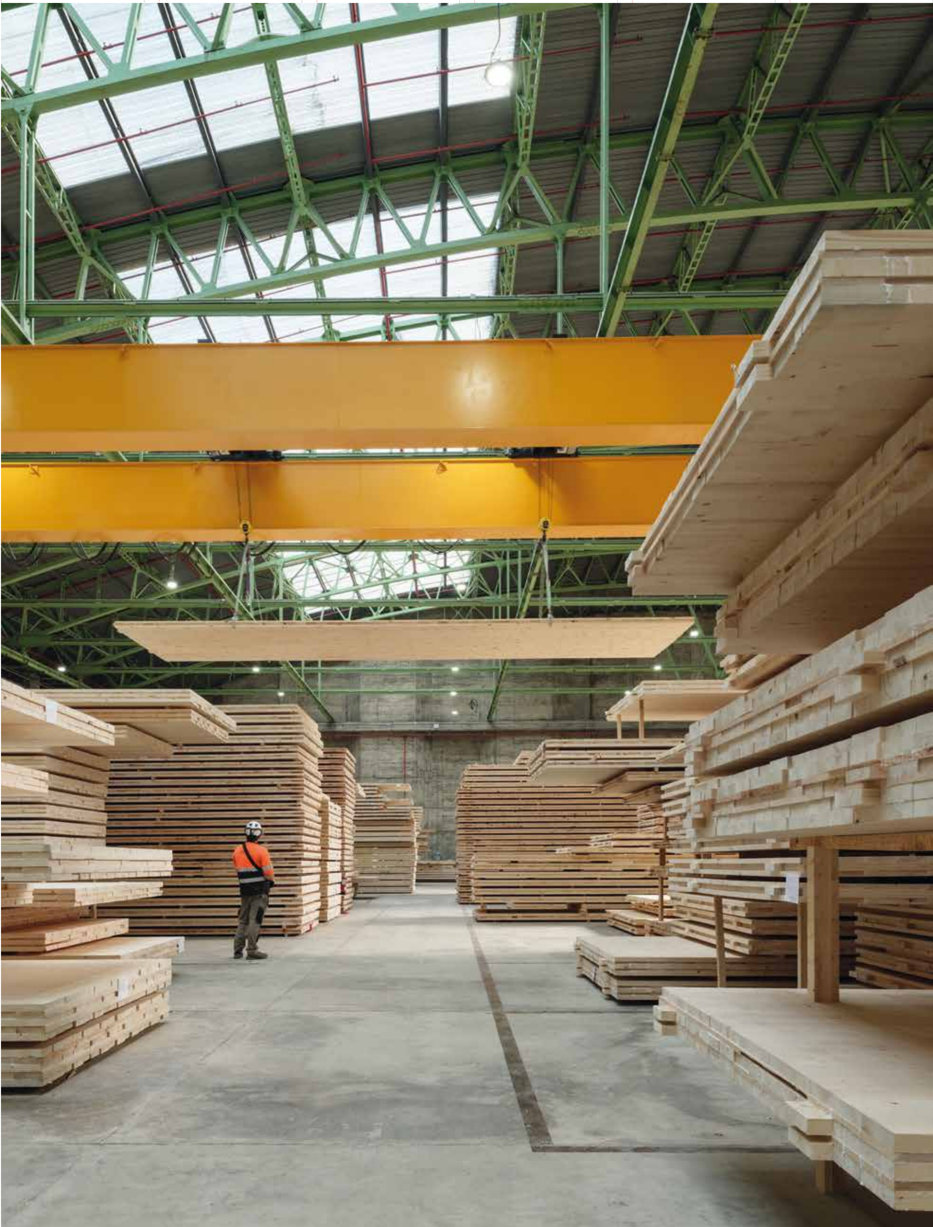
Almacén de paneles de madera contralaminada (CLT) en la planta de Egoín Albertia en Legutio (Araba). Foto: María Azkárte / Warehouse of cross-laminated timber panels (CLT) at Egoín Albertia's plant in Legutio (Araba). Photo: María Azkárte
